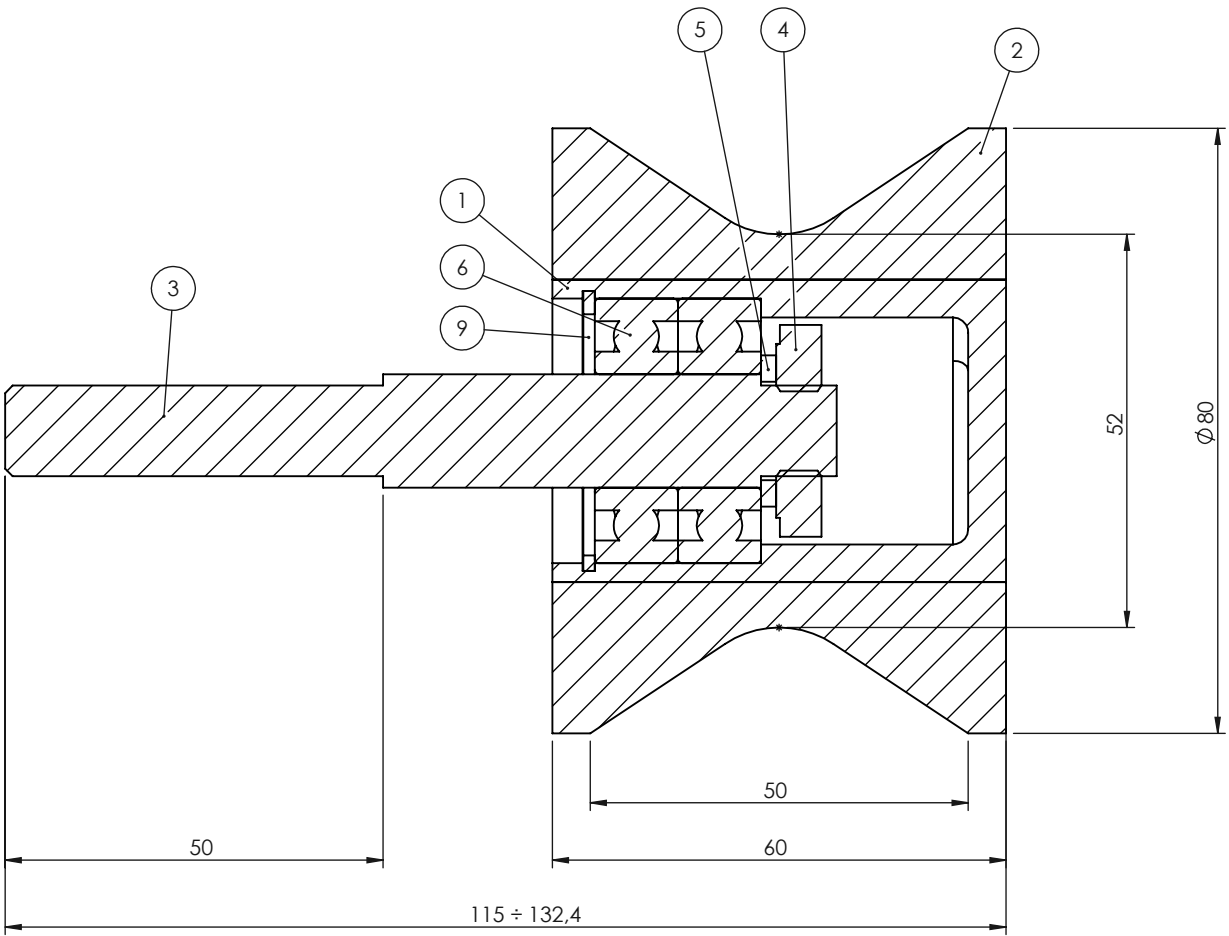
SEZIONE A-A
